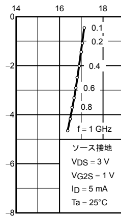
Y_{fs} - f 順伝達コンダクタンス g_{fs} (mS)
