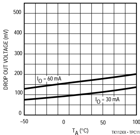
TK112XX · TPC11
