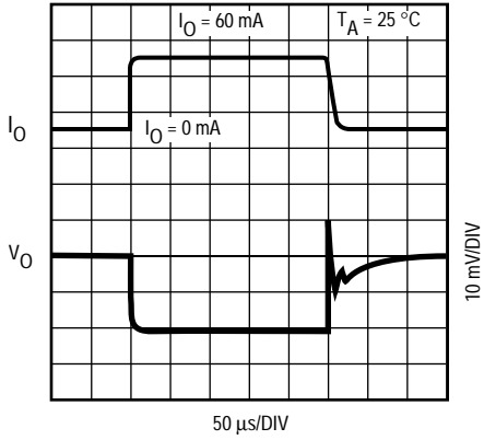
TK112XX · TPC07
