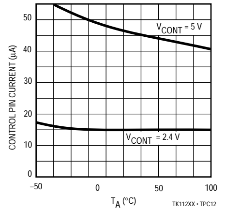
TK112XX · TPC12
