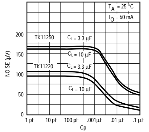
TK112XX · TPC09
